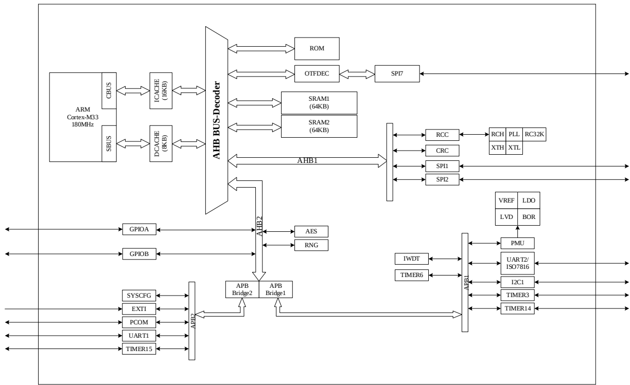
图 1-1 功能框图
