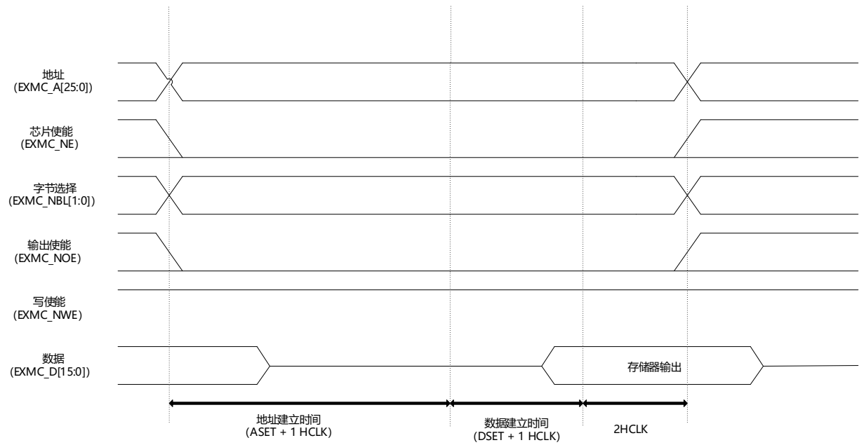
图 27-3 模式 1 读访问
