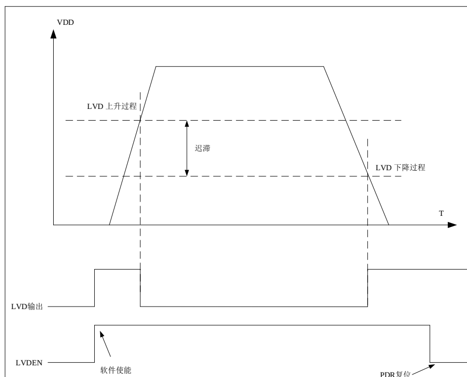
图 3-4 LVD 波形图
