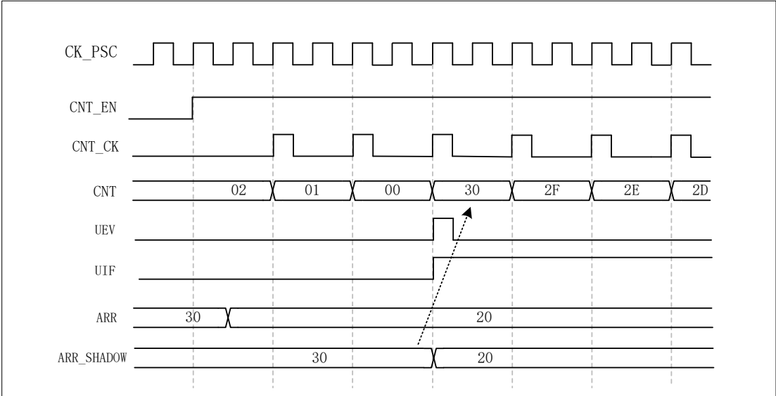
图 12-8 向上计数模式（使能自动重载预装载）
