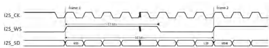
图 25-33 PCM 标准长帧同步模式时序图(DTLEN=00, CHLEN=0, CKPL=1)
