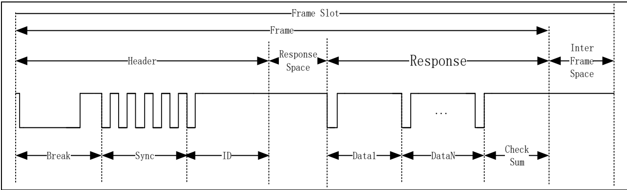
图 21-3 LIN 帧格式
