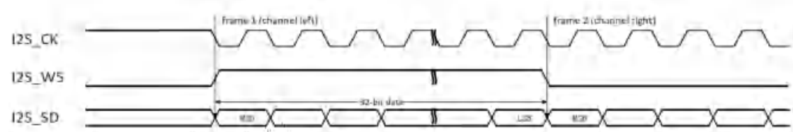
图 25-15 对齐标准时序图(DTLEN=10, CHLEN=1, CKPL=1)
