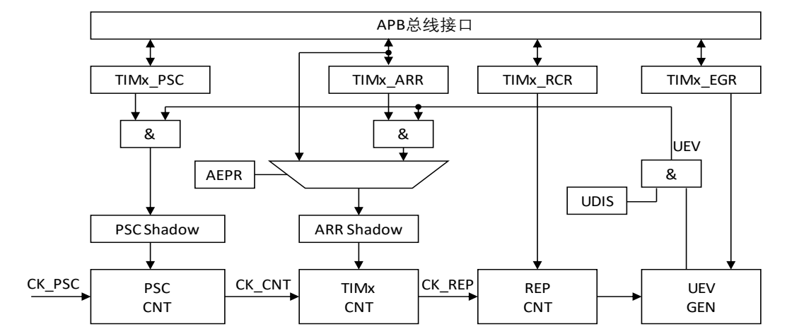
图 15-2 计数单元的结构
