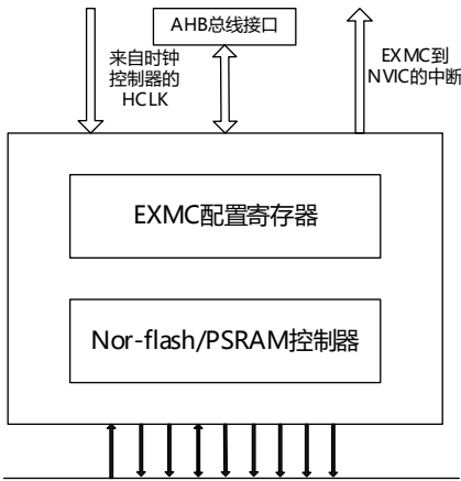
图 27-1 EXMC 结构框图
