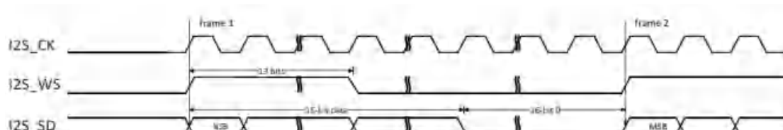
图 25-38 PCM 标准长帧同步模式时序图(DTLEN=00, CHLEN=1, CKPL=0)
