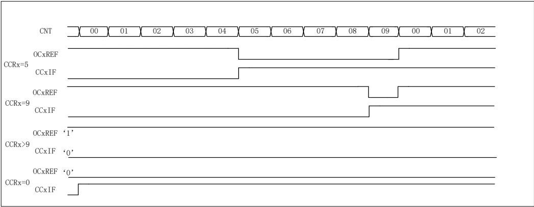
图 12-24 边沿对齐的 PWM 波形 (ARR=9)
