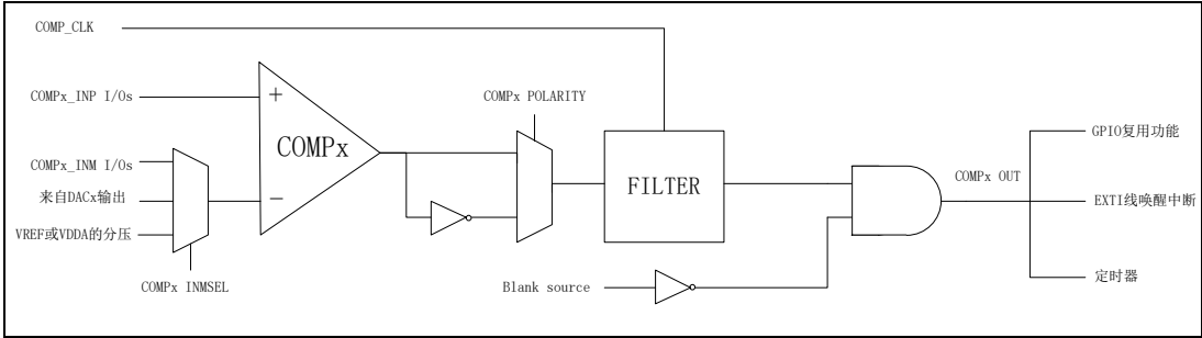
图 32-1 单个 COMP 结构框图
