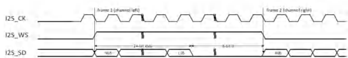
图 25-16 对齐标准时序图(DTLEN=01, CHLEN=1, CKPL=0)
