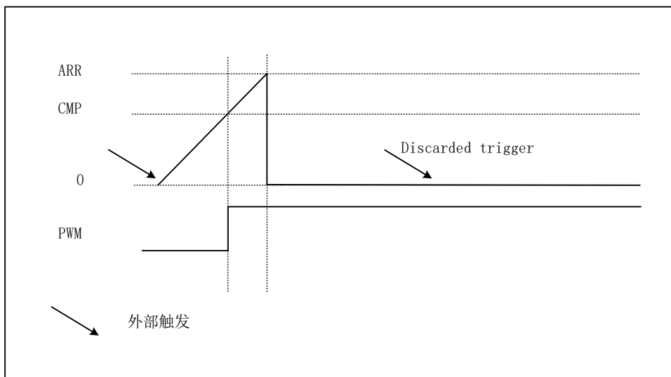
图 17-5 单次模式
