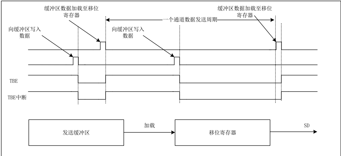
图 25-40 主发模式
