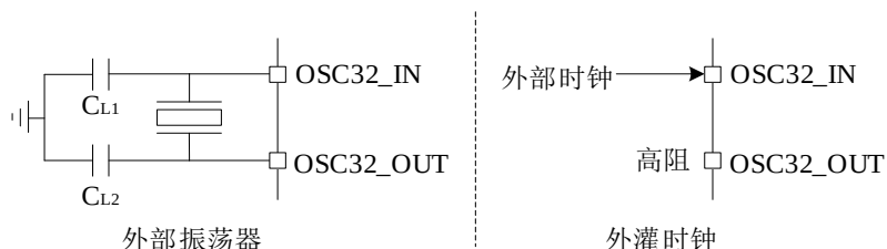
图 4-4 XTL 时钟
