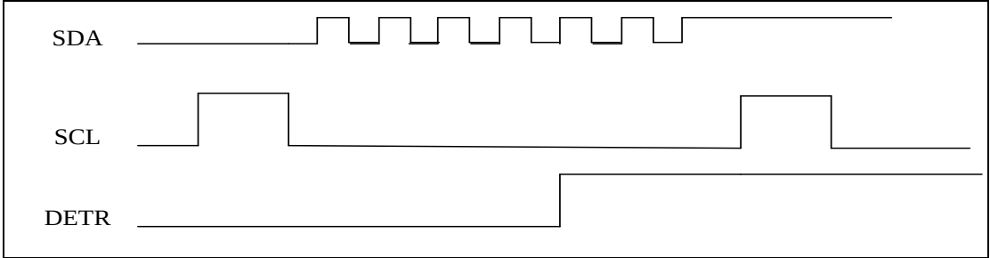
图 24-18 SDA 跳变检测图
