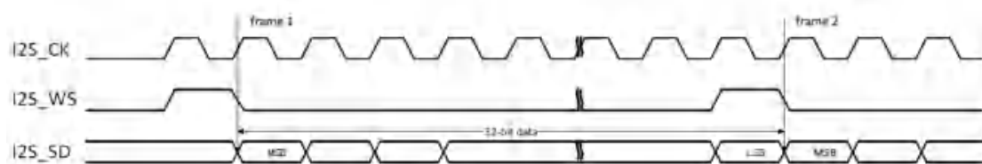
图 25-26 PCM 标准短帧同步模式时序图(DTLEN=10, CHLEN=1, CKPL=0)
