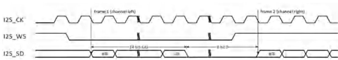
图 25-8 飞利浦标准时序图(DTLEN=01, CHLEN=1, CKPL=0)
