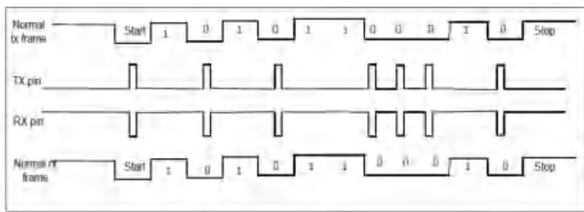
图 21-6 IrDA SIR 数据调制解调
