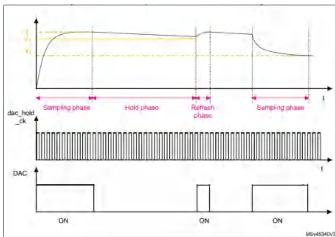
图 31-11 采样保持模式时序图
