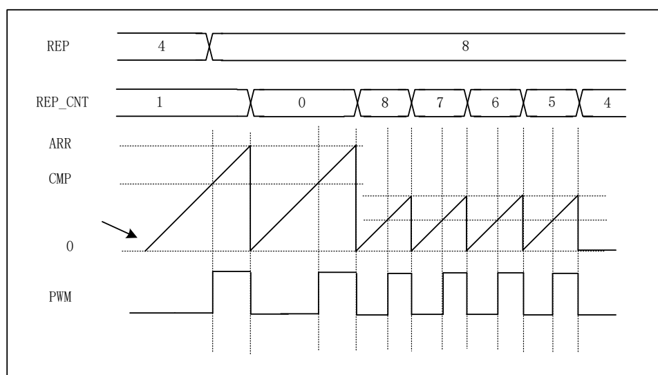
图 17-10 重复计数器
