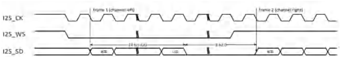
图 25-9 飞利浦标准时序图(DTLEN=01, CHLEN=1, CKPL=1)
