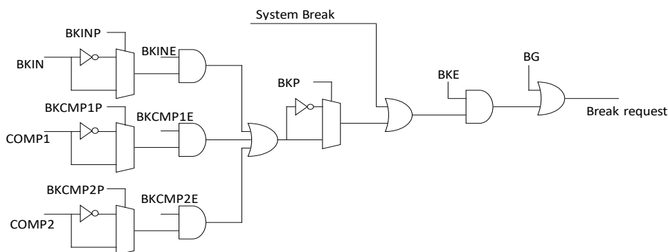
图 15-18 刹车
