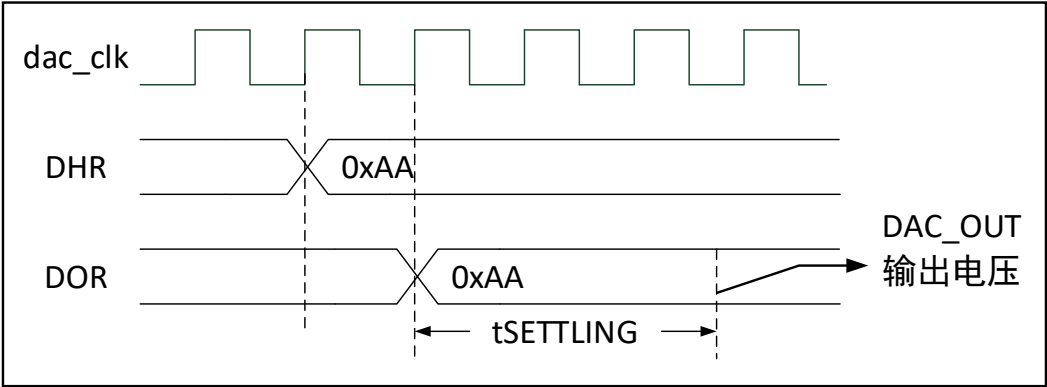
图 31-4 关闭触发 (TEN=0) 时的转换时序图
