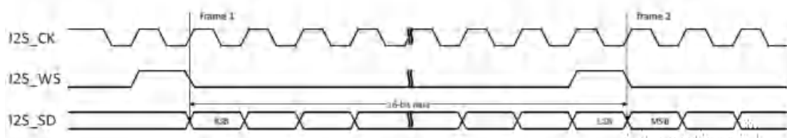
图 25-25 PCM 标准短帧同步模式时序图(DTLEN=00, CHLEN=0, CKPL=1)
