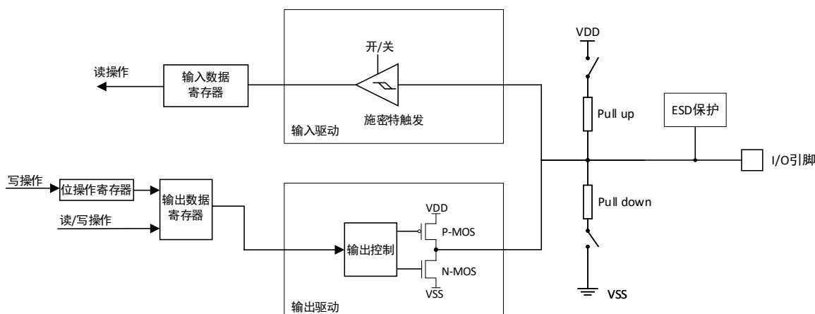
图 8-3 输出配置
