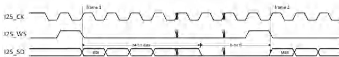
图 25-29 PCM 标准短帧同步模式时序图(DTLEN=01, CHLEN=1, CKPL=1)
