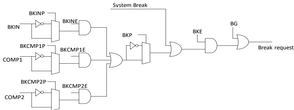
图 16-12 刹车
