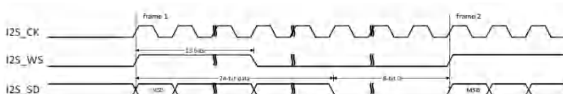
图 25-36 PCM 标准长帧同步模式时序图(DTLEN=01, CHLEN=1, CKPL=0)
