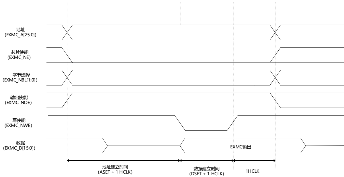
图 27-4 模式 1 写访问
