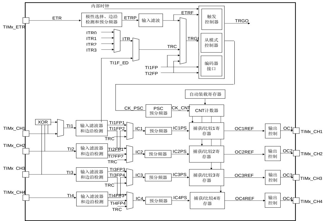
图 13-1 通用定时器框图
