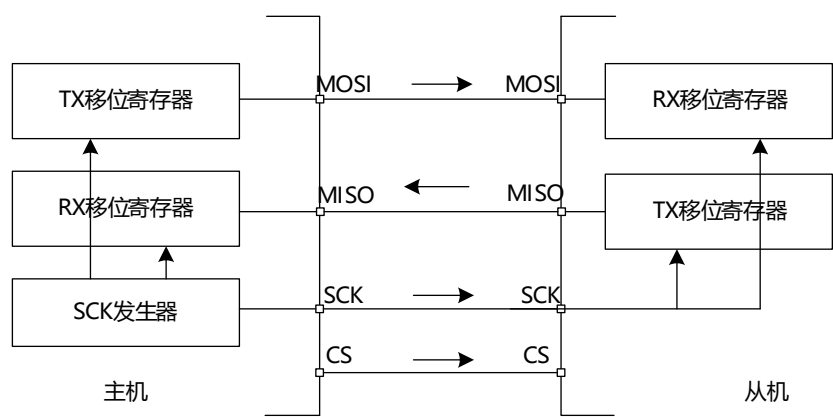
图 23-8 SPI 全双工通信
