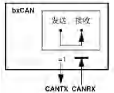
图 26-5 环回静默模式示意图
