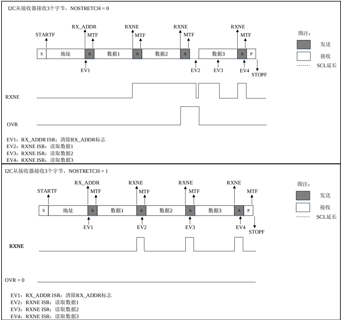
图 24-12 I2C 从模式接收时序
