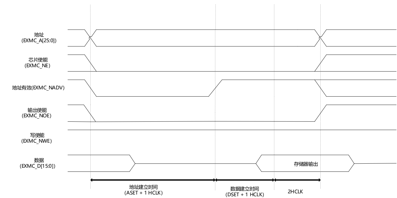
图 27-7 模式 2 读访问
