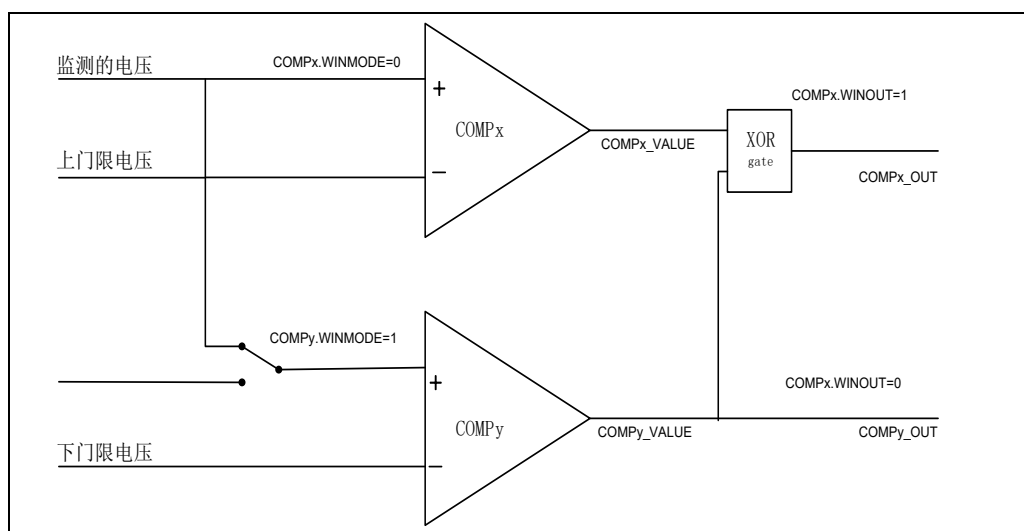
图 32-7 窗口比较器
