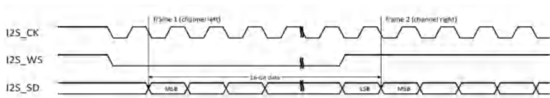
图 25-6 飞利浦标准时序图(DTLEN=10, CHLEN=1, CKPL=0)
