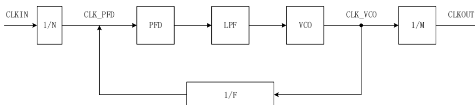
图 4-5 PLL 功能框图
