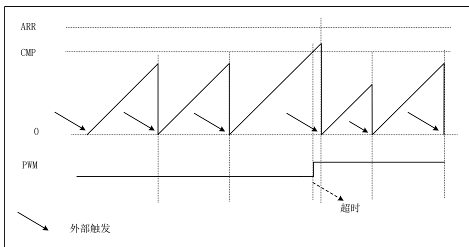
图 17-7 超时
