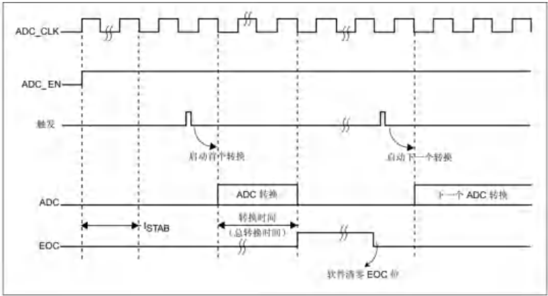
图 30-2 ADC 转换时序图
