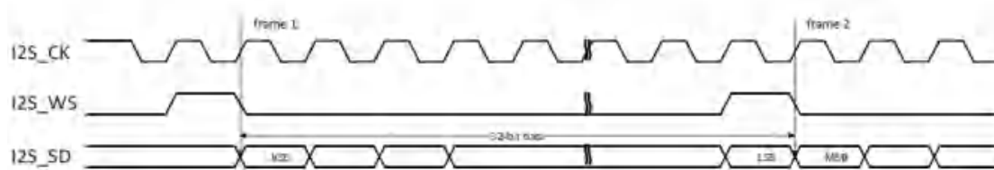
图 25-27 PCM 标准短帧同步模式时序图(DTLEN=10, CHLEN=1, CKPL=1)
