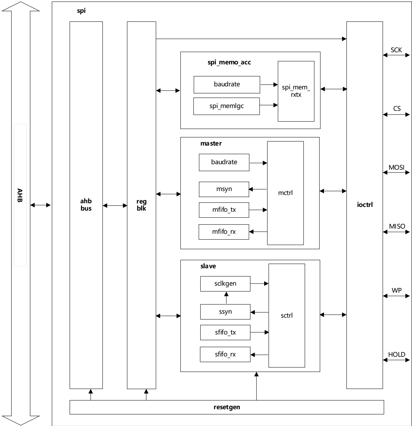
图 23-1 SPI 框图
