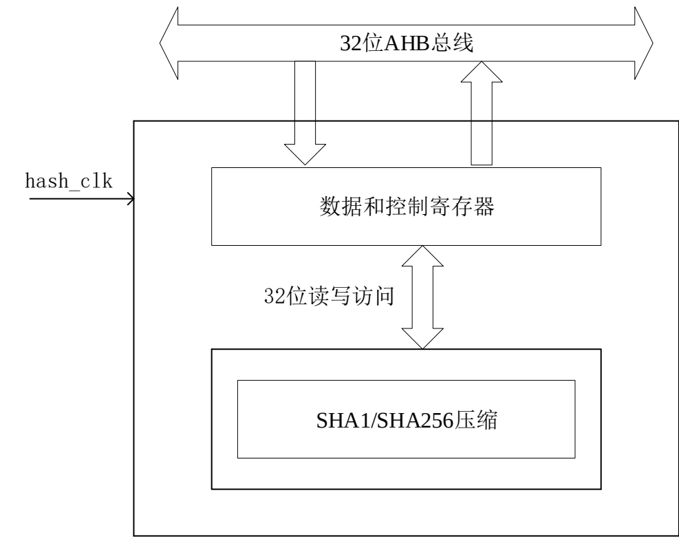
图 38-1 SHA 结构框图
