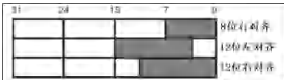
图 31-2 DAC 单通道模式的数据寄存器
