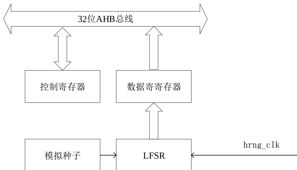
图 37-1 HRNG 框图
