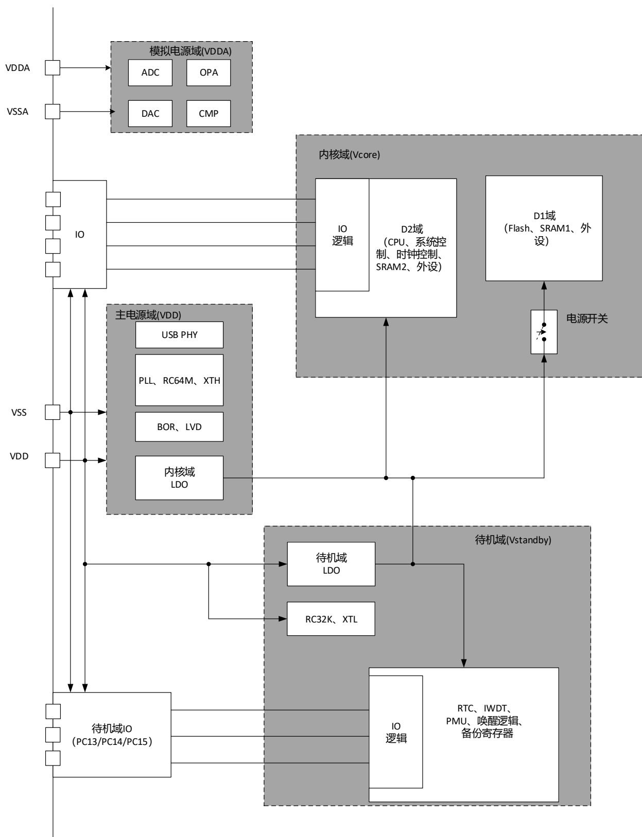
图 3-1 电源管理结构框图
