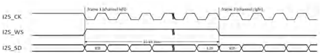
图 25-13 对齐标准时序图(DTLEN=00, CHLEN=0, CKPL=1)
