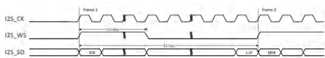
图 25-34 PCM 标准长帧同步模式时序图(DTLEN=10, CHLEN=1, CKPL=0)
