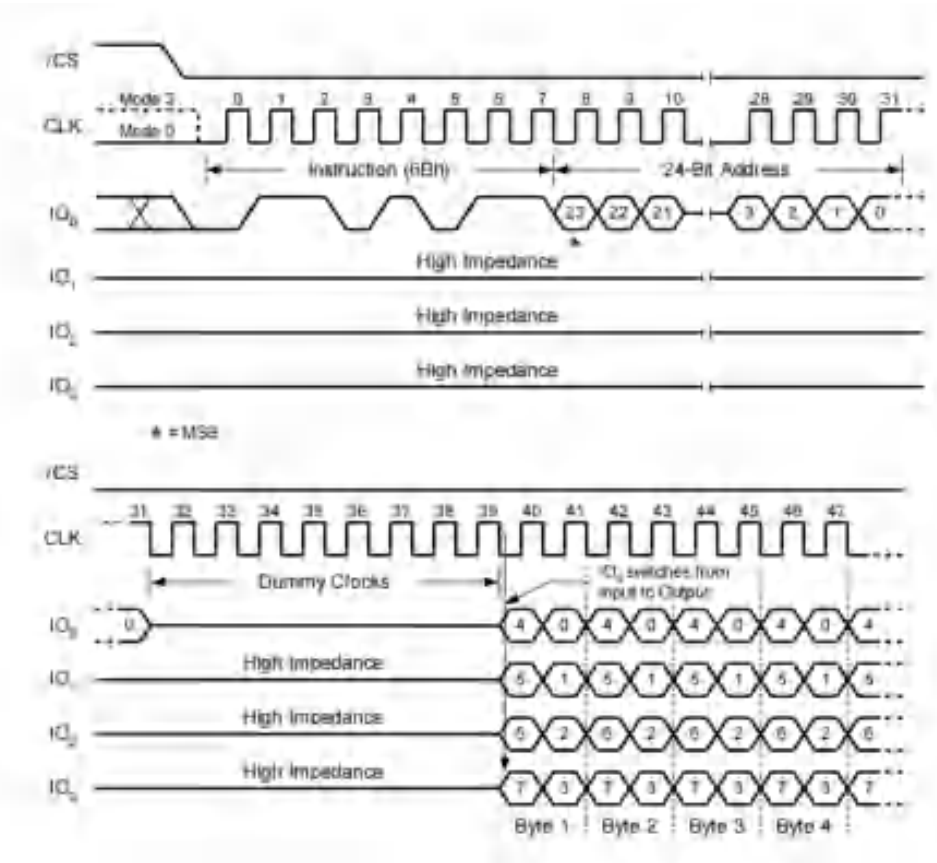
图 23-14 SPI 访问存储器命令序列
