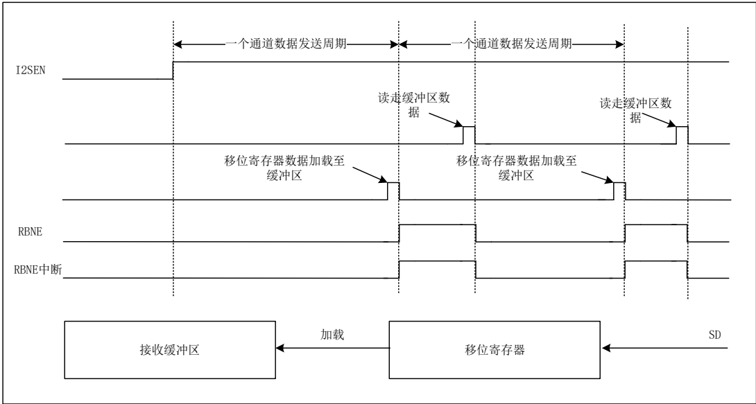
图 25-41 主收模式
