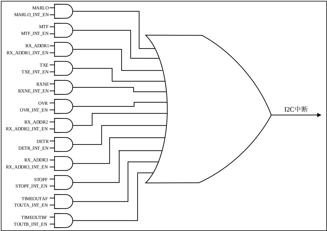
24-24 I2C 中断映射图图
