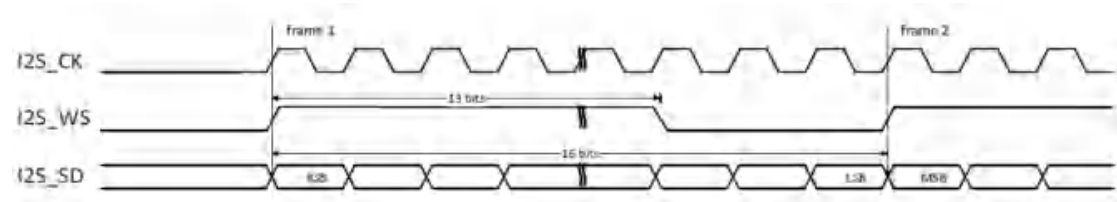
图 25-32 PCM 标准长帧同步模式时序图(DTLEN=00, CHLEN=0, CKPL=0)
