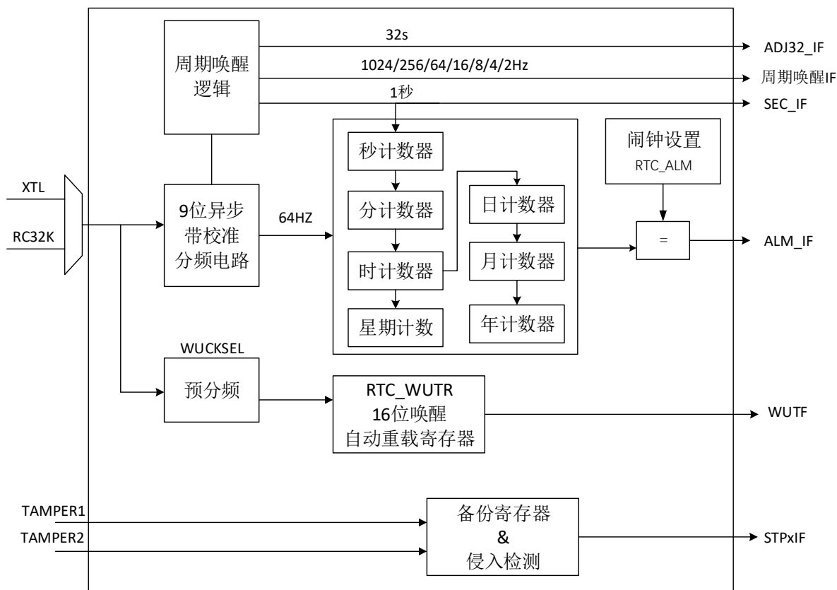
图 20-1 RTC 内部结构框图
