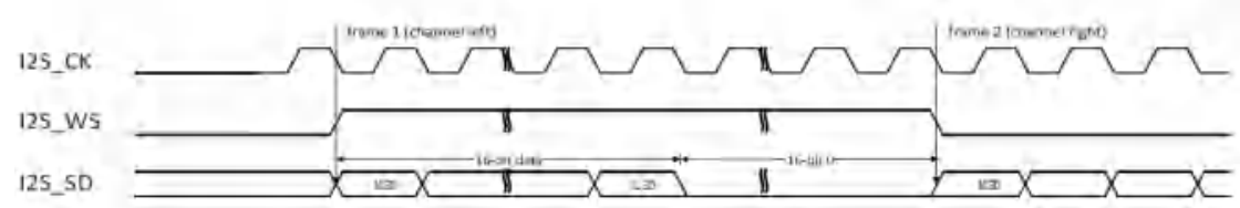
图 25-18 对齐标准时序图(DTLEN=00, CHLEN=1, CKPL=0)
