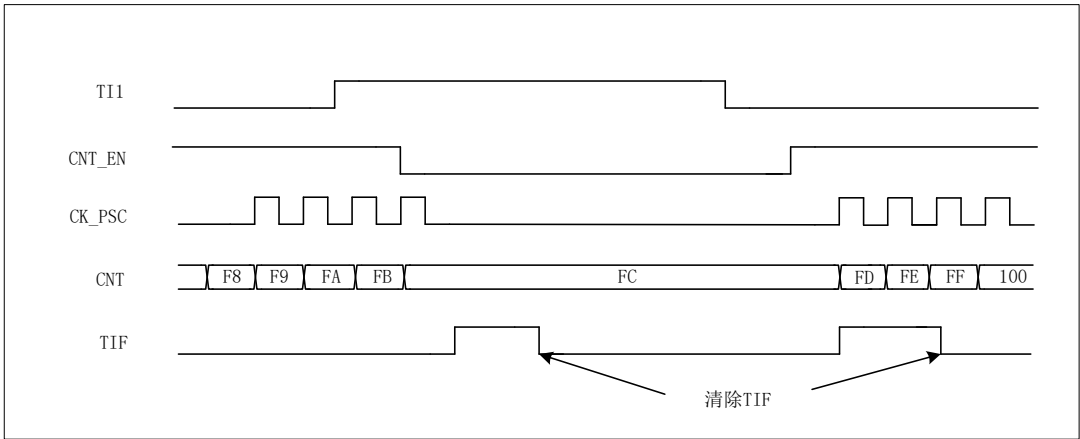
图 15-22 门控模式下的控制电路
