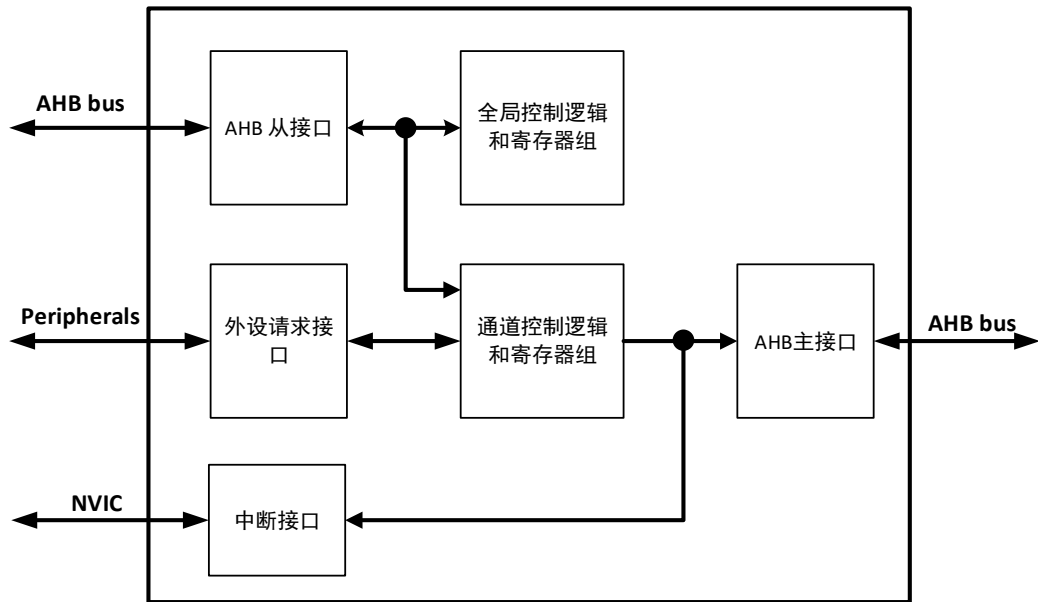
图 9-1 DMA 框图
