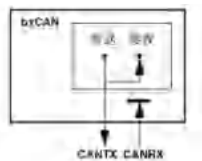
图 26-4 环回模式示意图
