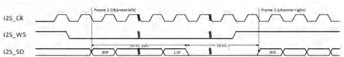
图 25-10 飞利浦标准时序图(DTLEN=00, CHLEN=1, CKPL=0)
