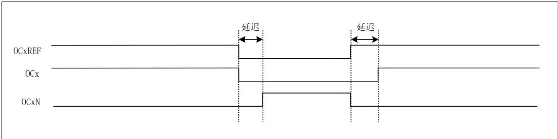
图 16-10 死区波形延迟大于负脉冲
