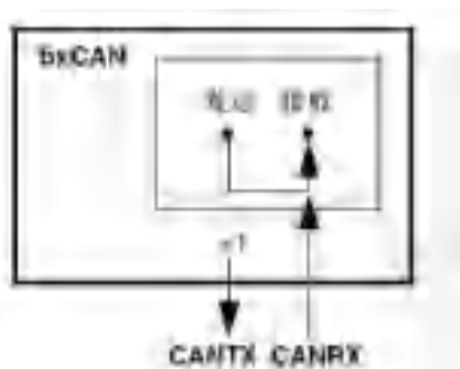
图 26-3 静默模式示意图
