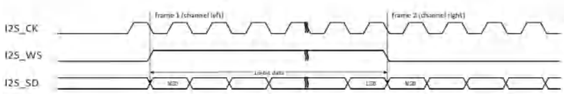
图 25-12 MSB 对齐标准时序图(DTLEN=00, CHLEN=0, CKPL=0)
