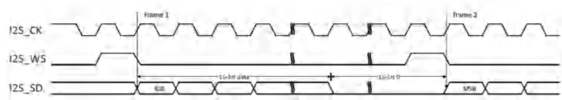
图 25-31 PCM 标准短帧同步模式时序图(DTLEN=00, CHLEN=1, CKPL=1)
