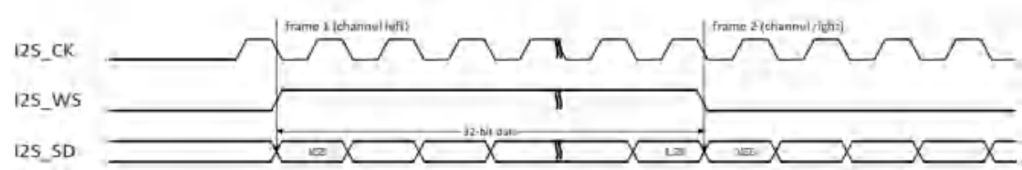
图 25-14 对齐标准时序图(DTLEN=10, CHLEN=1, CKPL=0)
