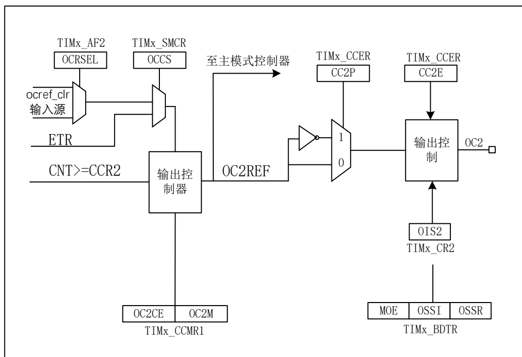
图 15-12 捕获/比较通道的输出部分(通道 2)
