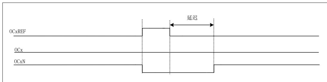
图 15-17 死区波形延迟大于正脉冲
