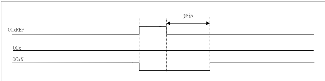
图 16-11 死区波形延迟大于正脉冲
