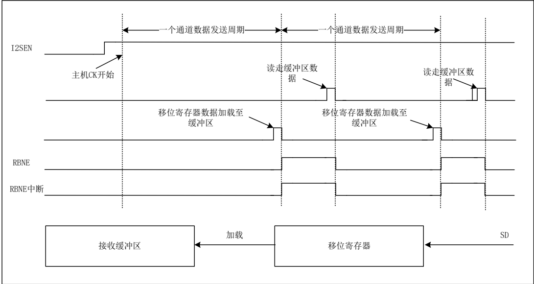
图 25-44 从收模式
