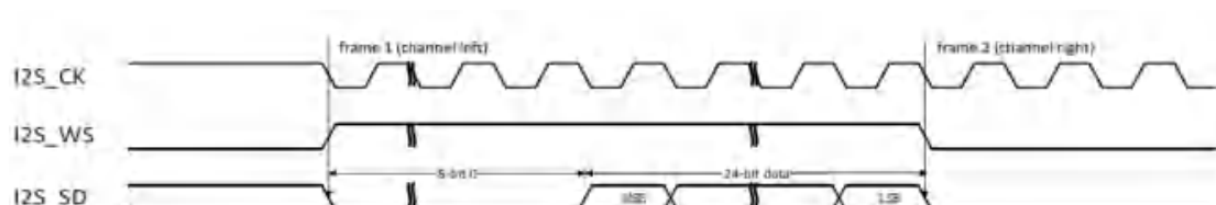
图 25-21 LSB 对齐标准时序图(DTLEN=01, CHLEN=1, CKPL=1)
