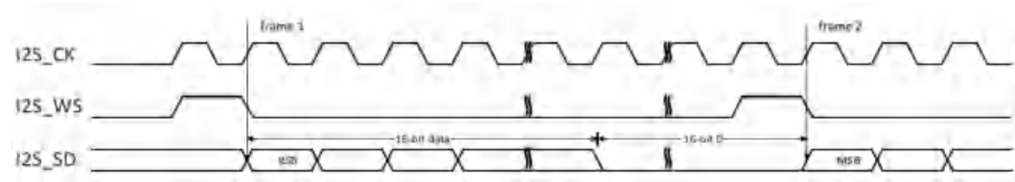
图 25-30 PCM 标准短帧同步模式时序图(DTLEN=00, CHLEN=1, CKPL=0)
