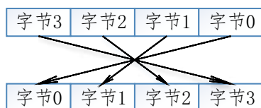
图 35-6 SWAP 模式
