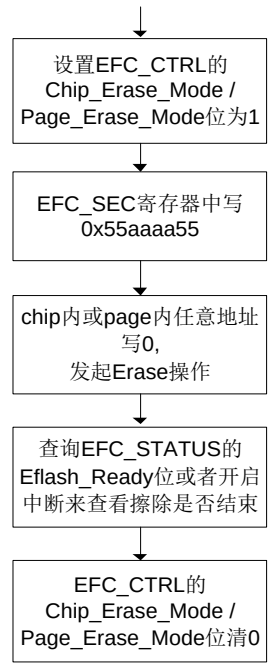
图 10-5 Erase 操作流程
