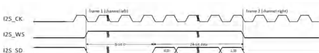
图 25-20 对齐标准时序图(DTLEN=01, CHLEN=1, CKPL=0)
