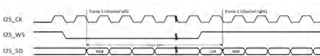
图 25-5 飞利浦标准时序图(DTLEN=00, CHLEN=0, CKPL=1)
