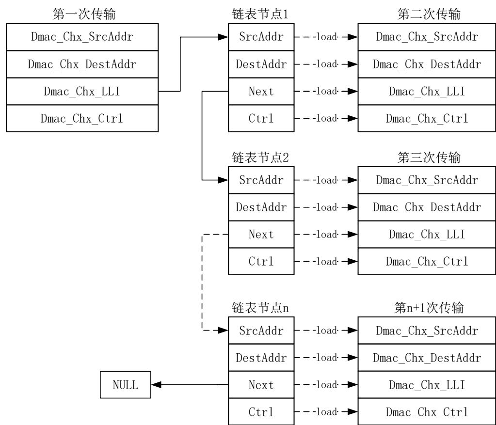
图 9-2 链表结构示意图
