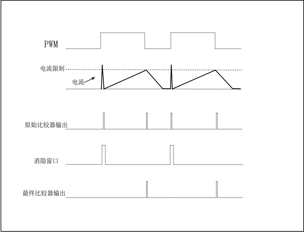
图 32-6 比较器输出消隐
