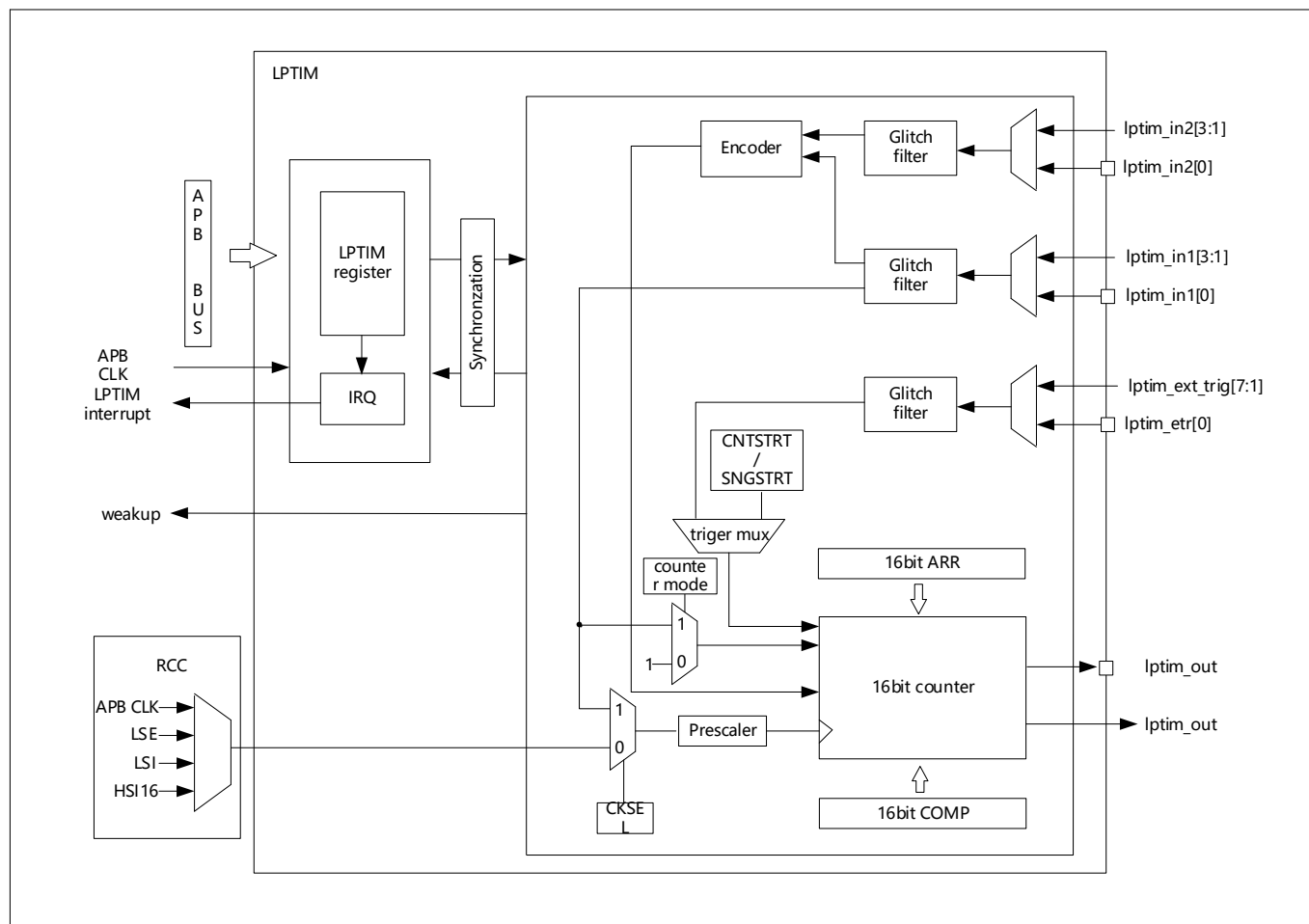
图 17-1 LPTIM 框图
