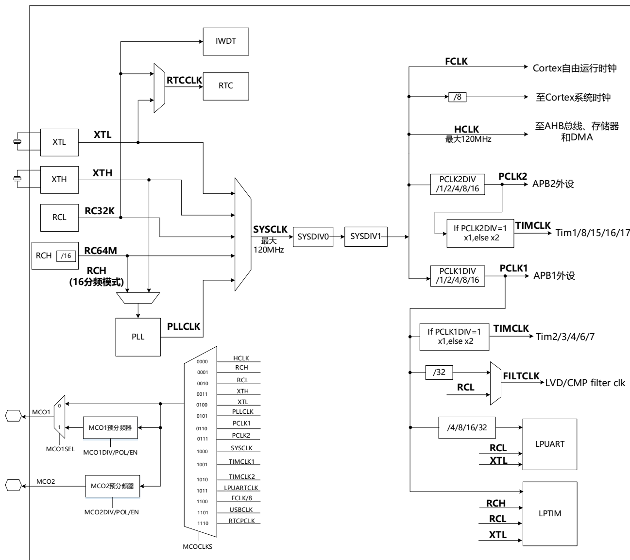
图 4-2 时钟结构图
