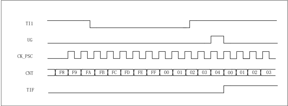
图 15-21 复位模式下的控制电路
