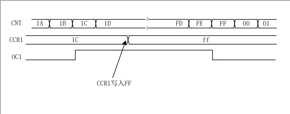
图 15-14 输出比较模式，翻转 OC1
