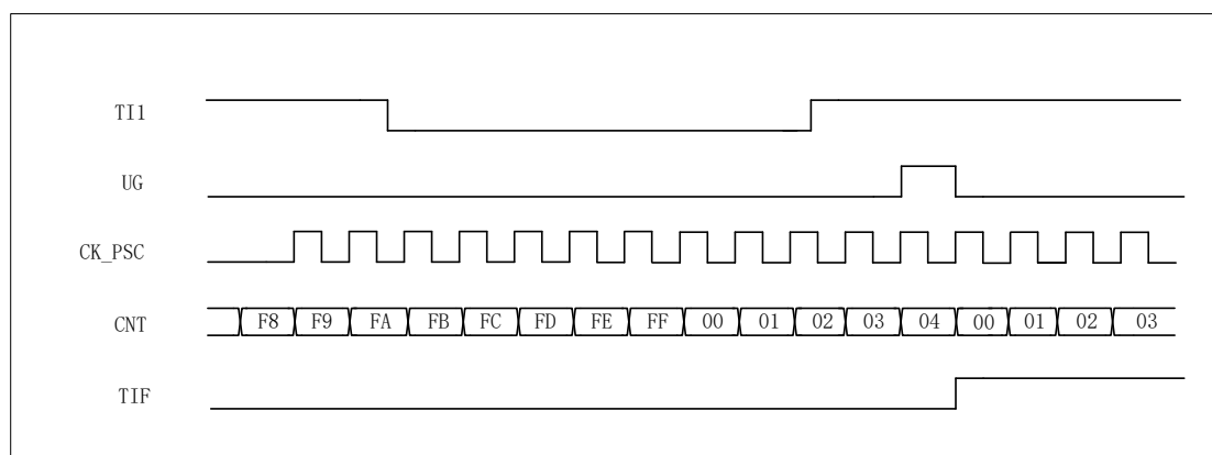
图 12-35 复位模式下的控制电路
