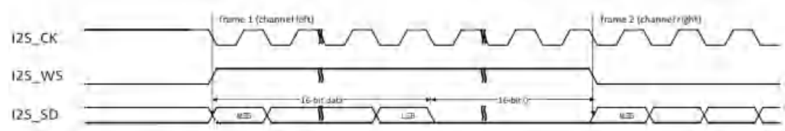
图 25-19 对齐标准时序图(DTLEN=00, CHLEN=1, CKPL=1)
