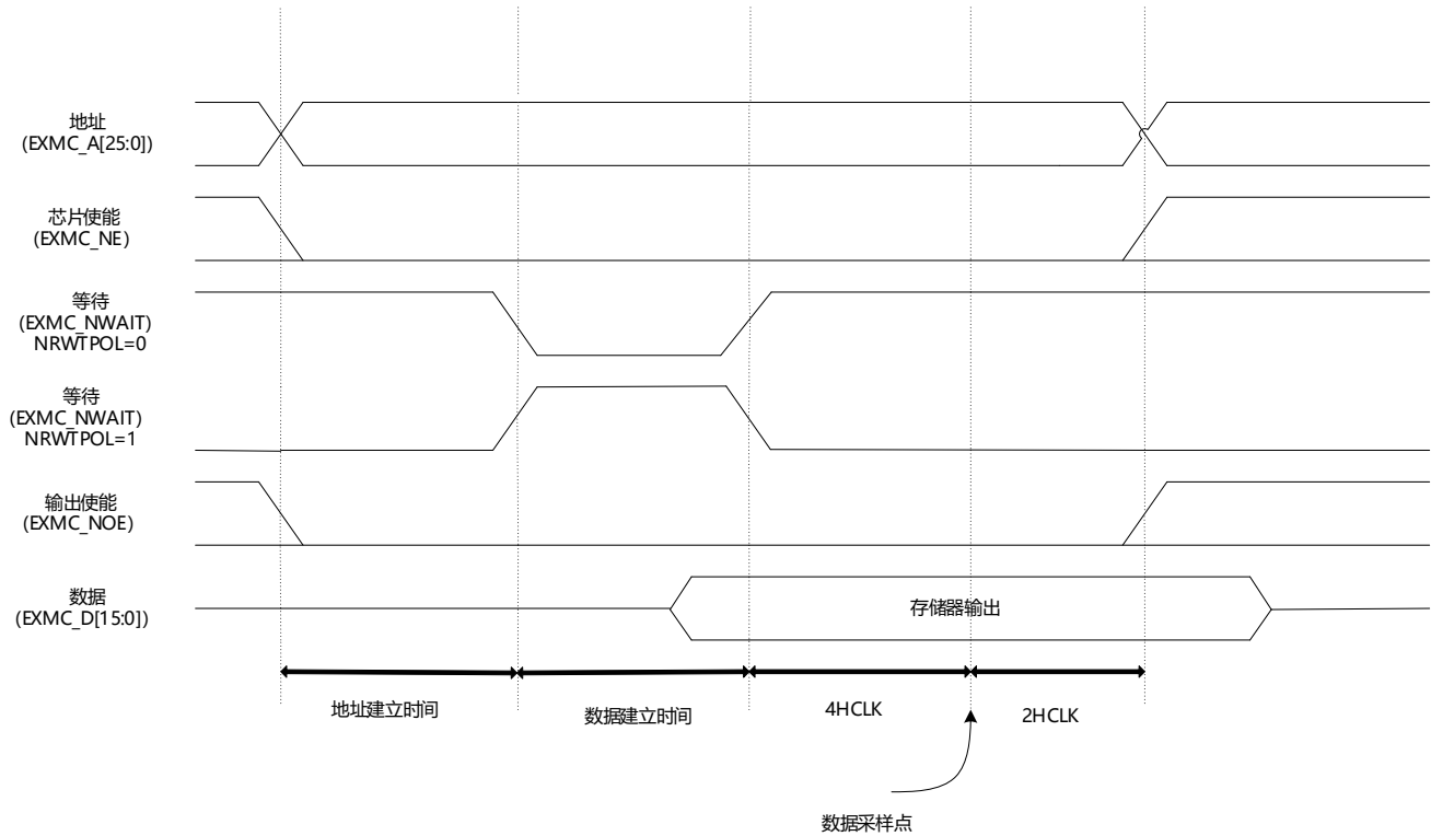
图 27-16 异步等待有效时的读时序
