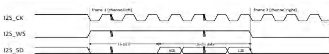
图 25-23 LSB 对齐标准时序图(DTLEN=00, CHLEN=1, CKPL=1)
