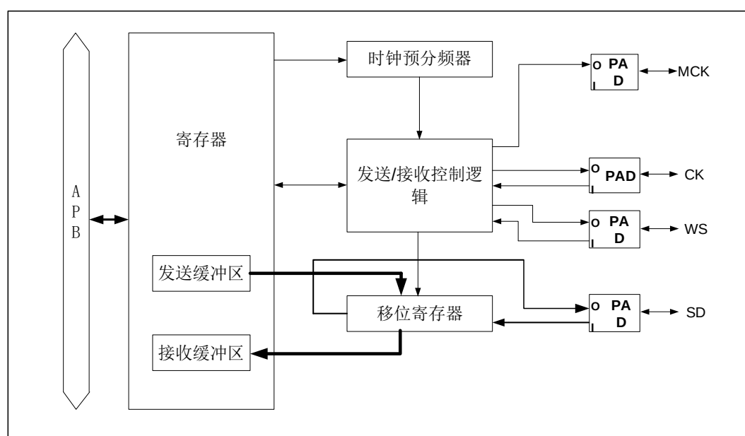
图 25-1 I2S 框图
