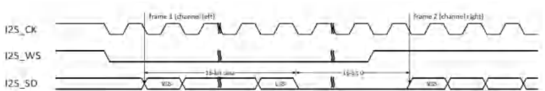
图 25-11 飞利浦标准时序图(DTLEN=00, CHLEN=1, CKPL=1)
