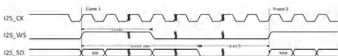
图 25-37 PCM 标准长帧同步模式时序图(DTLEN=01, CHLEN=1, CKPL=1)
