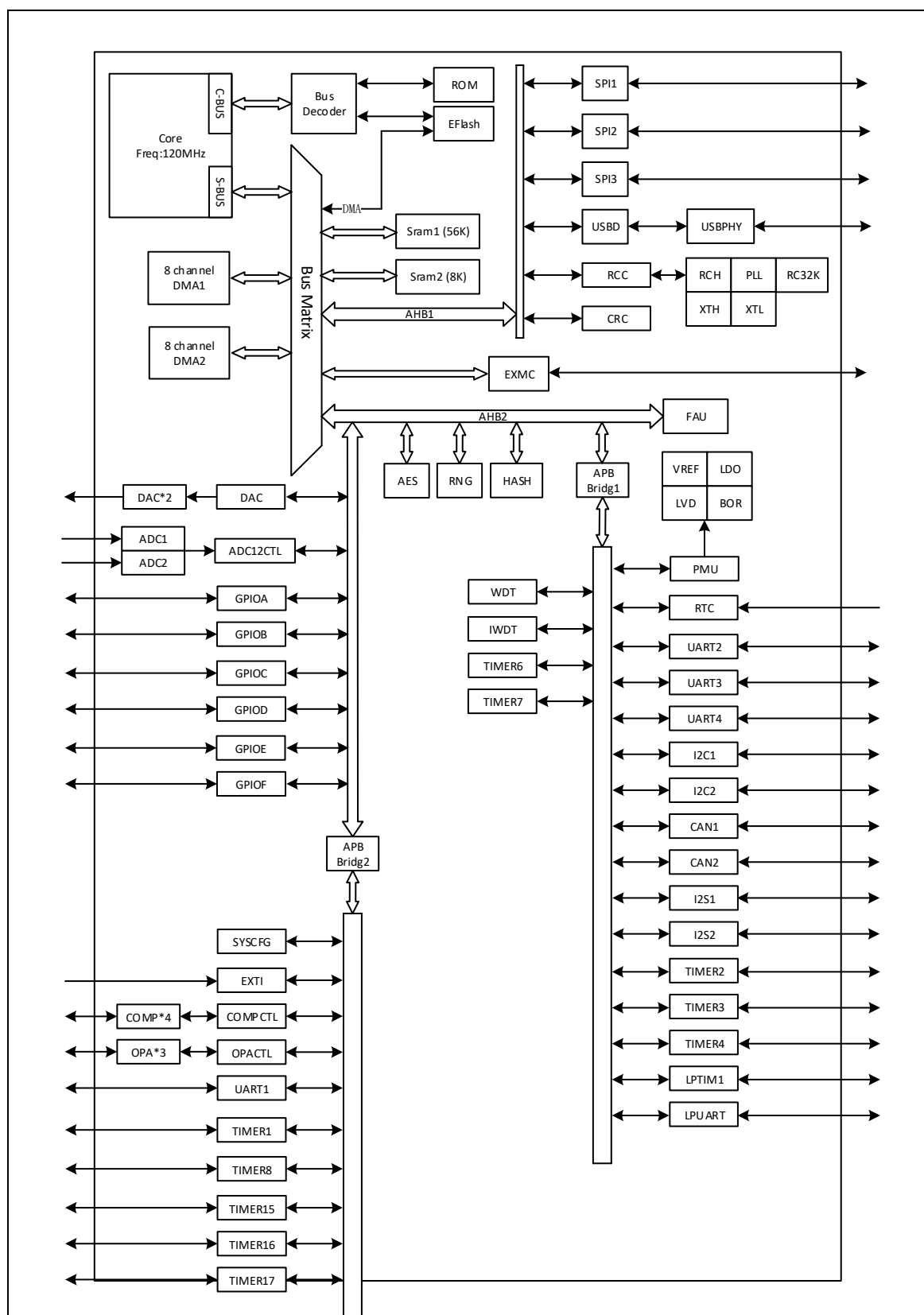
图 2-2 系统架构
