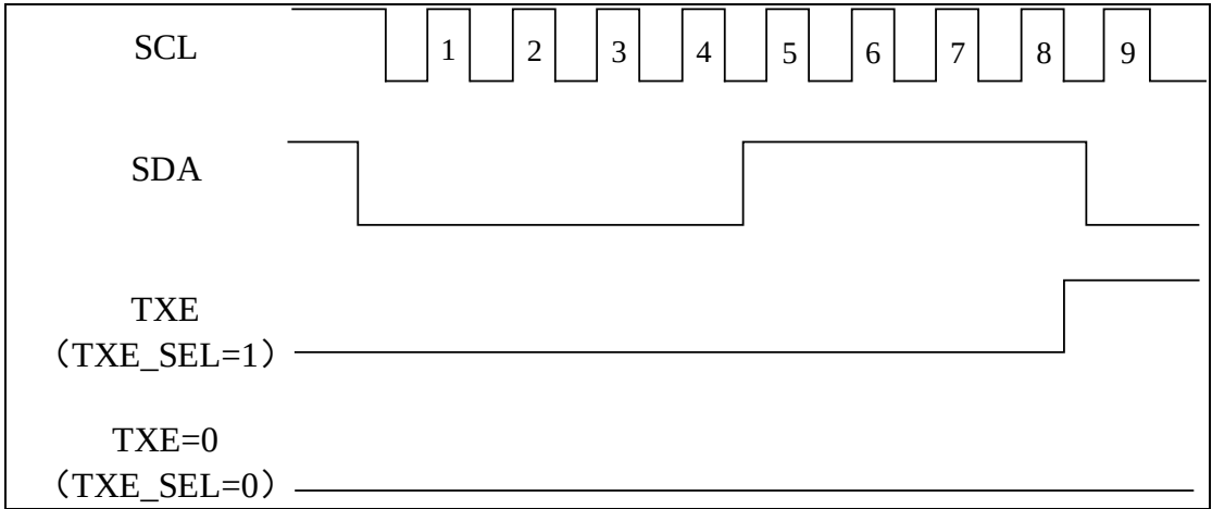
图 24-20 TXE 状态变化
