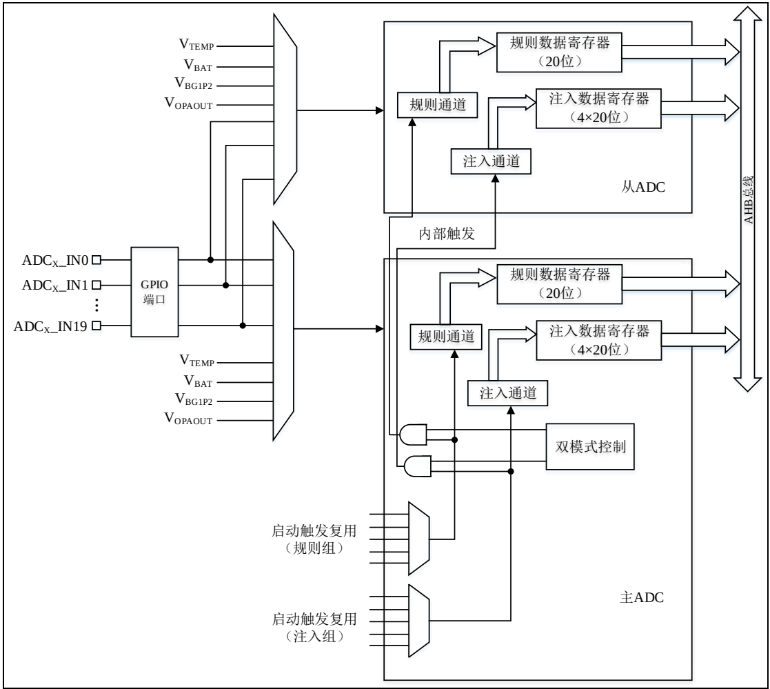
图 30-6 双 ADC 模式
