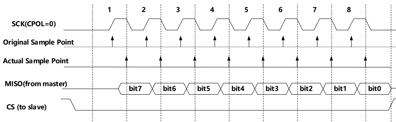
图 23-11 移位采样示意图 (CPOL=0, CPHA=0, MSB)
