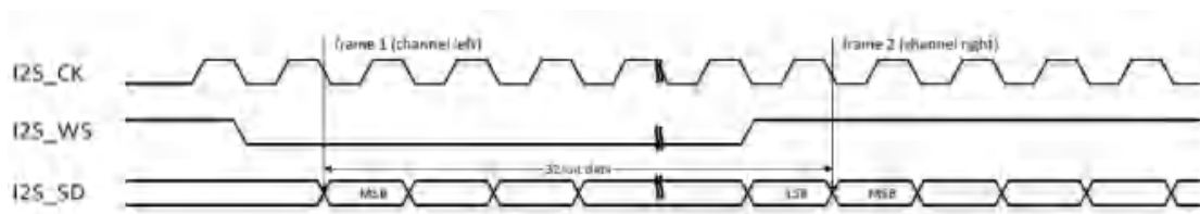
图 25-7 飞利浦标准时序图(DTLEN=10, CHLEN=1, CKPL=1)
