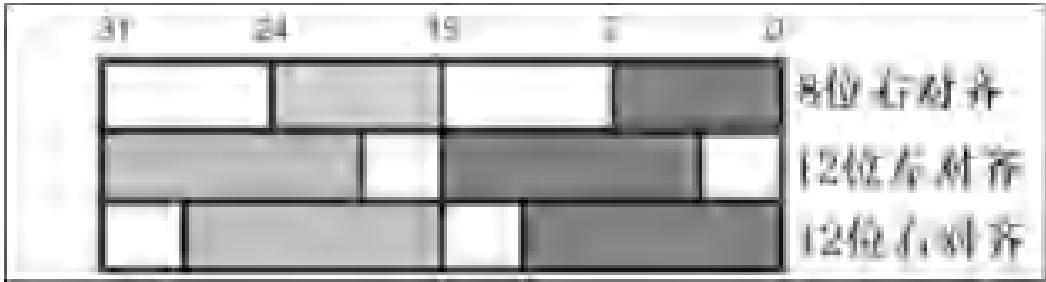
图 31-3 DAC 双通道模式的数据寄存器
