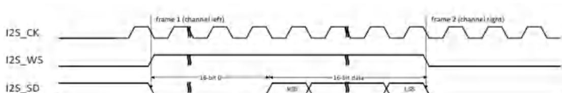
图 25-22 LSB 对齐标准时序图(DTLEN=00, CHLEN=1, CKPL=0)
